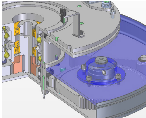
TRASMISSIONE CON INGRANAGGI TEMPERATI. Planetario al 100% in metallo temperato e senza cinghia.
